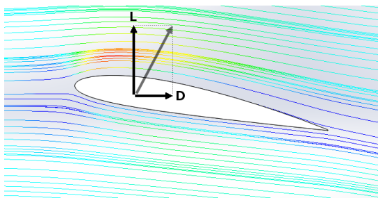
Figur 3: Hastighedsfordeling ved strømning omkring et vingeprofil. Den resulterende aerodynamiske kraft består af opdrift ( L ) og modstand ( D ).
