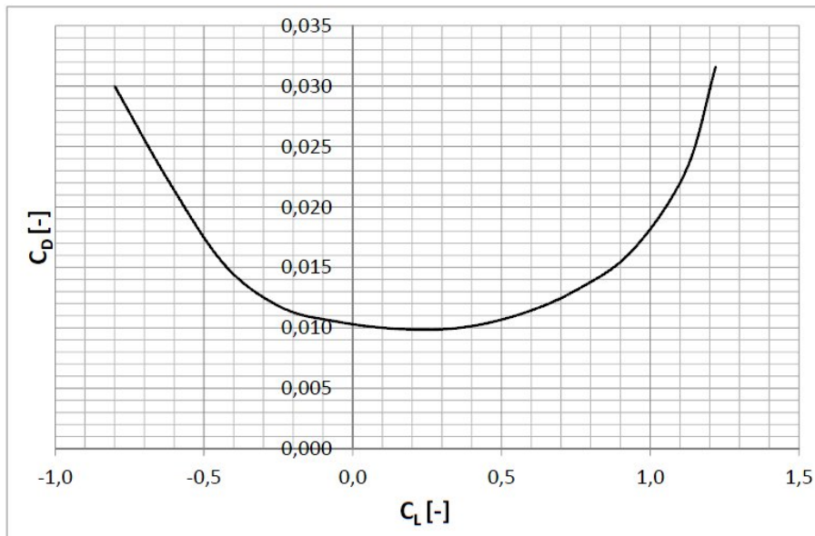
Figur 5: Dragkurve som funktion af liftkoefficienten. Her vist for et NACA 23012 profil.
